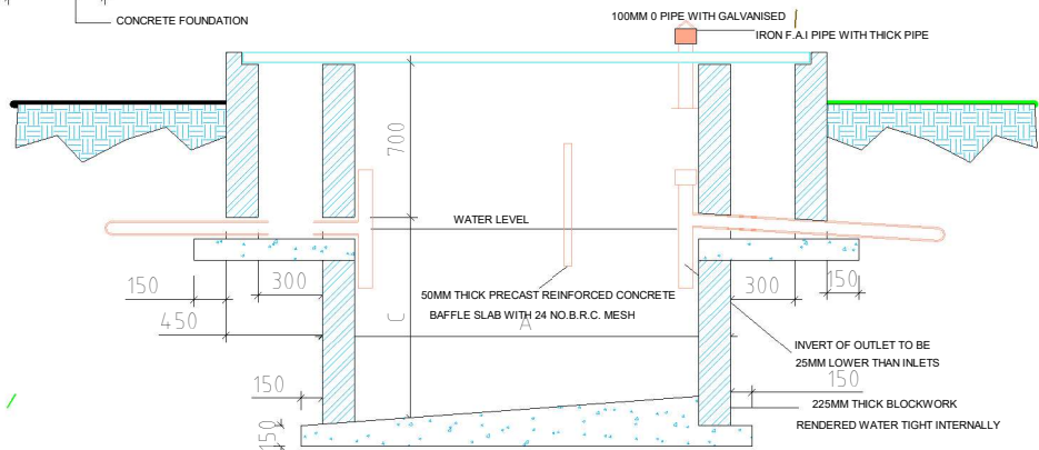
LONGITUDINAL SECTION A-A
